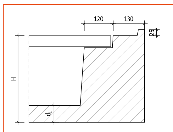
Detail-C1
