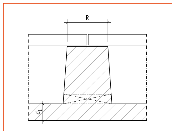
Detail-D
